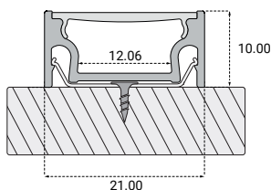
montaż nawierzchniowy
