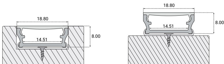
montaż wpustowy
