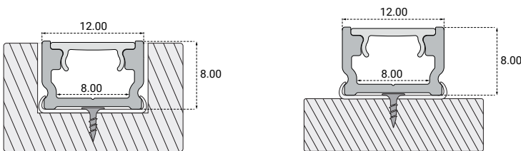
Installation encastrée
